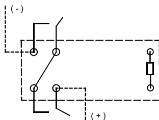
接线图
