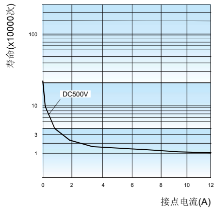
阻性电耐久性曲线图
