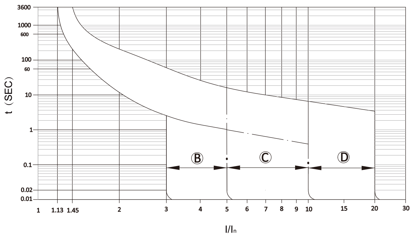
脱扣特性B、C、D
